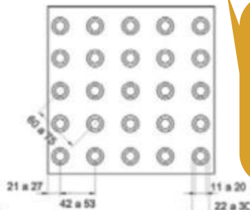
FIGURA 1 – SINALIZAÇÃO TÁTIL DE ALERTA – MODULAÇÃO DO PISO
